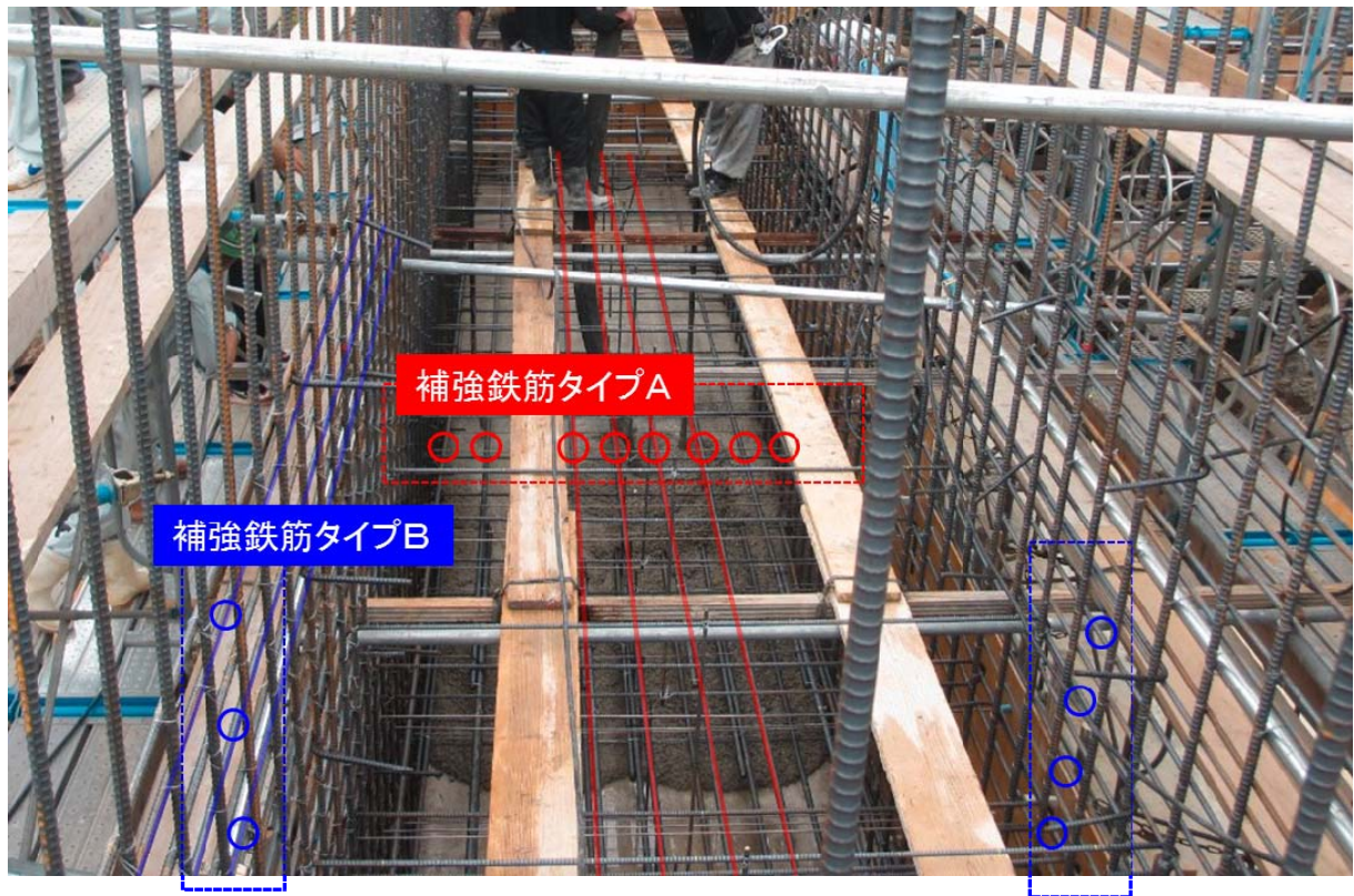
図 3.3.11 補強鉄筋配置状況図
