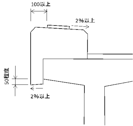
地覆部
