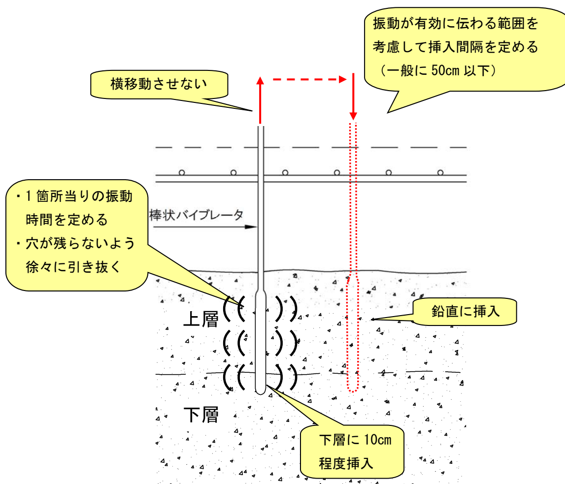
図 3.2.2 締固め時留意点の概要図
