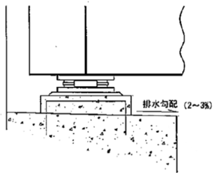
橋座面
